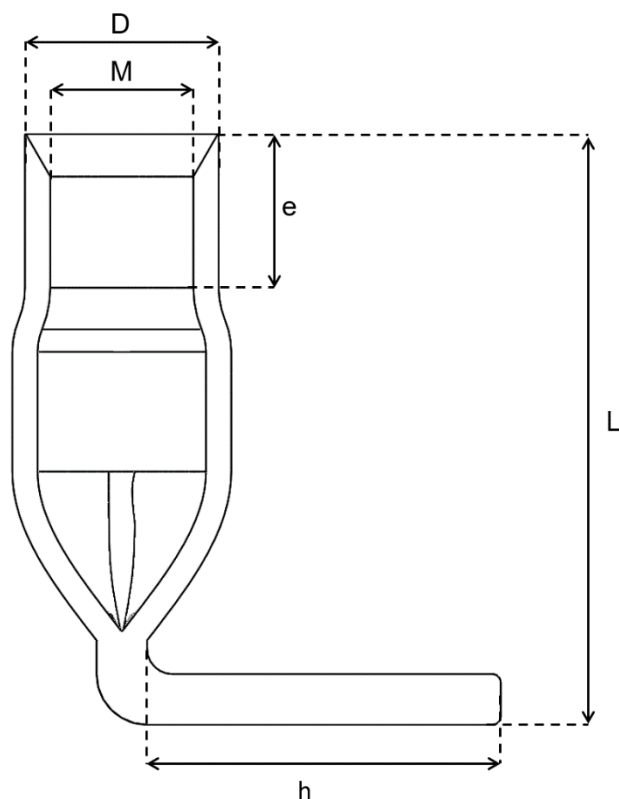
Figur 6 Befæstigelses insert med vinkel ende skitse.
