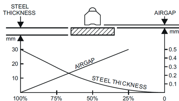
POWERTEXi tõstemagnet nimikoormus 300 kg
