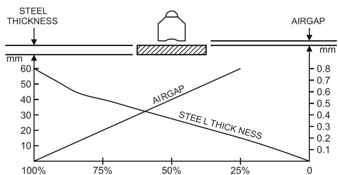
POWERTEX potencia nominal 2 t
