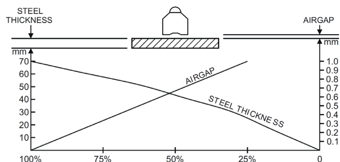
POWERTEX puissance nominale 2 t
