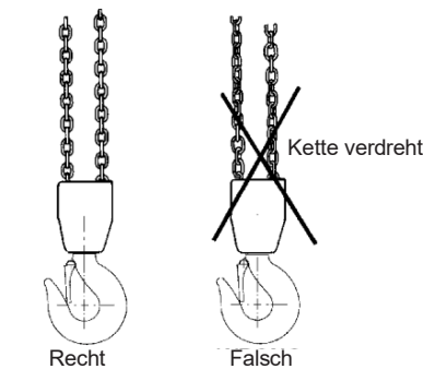
Abb. 3 Die Kette darf nicht verdreht sein
