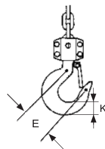
Imag. 4: Gancho de carga
