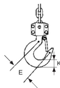
Fig. 4 Lastkrog
