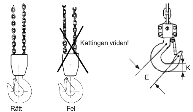
Fig 3 Kättingen får ej vara vriden
