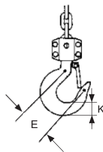
Kuva 4. Kuormakoukku
