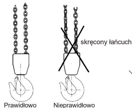
Rys. 3 Łańcuch nie powinien być skręcony
