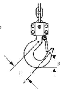
4. attēls. Kravas āķis
