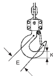
Joonis 4 Tõstekonks
