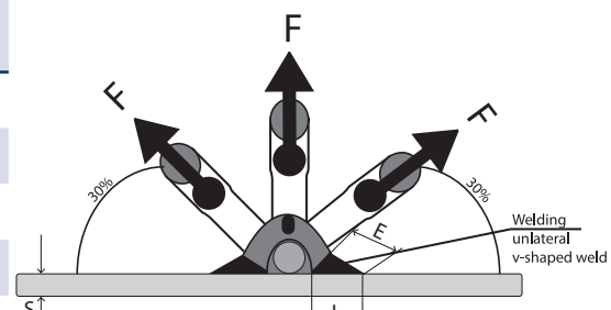
Lassen en gebruik van schematisch diagram van D-ring
