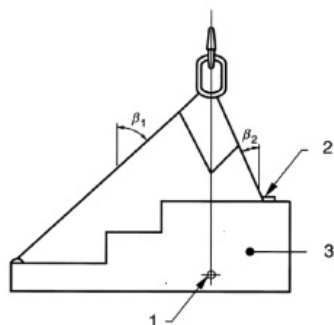
1. centre de gravité 2. tension élevée dans ce brin 3. charge P
