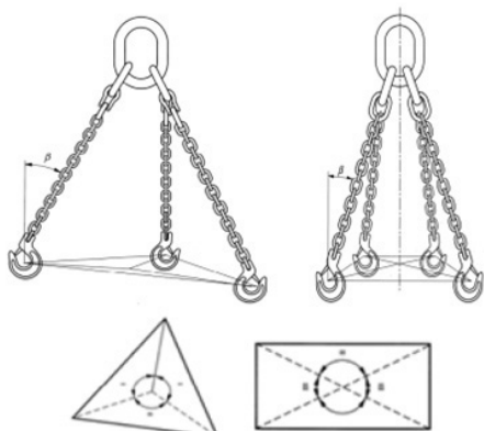
Symetria obciążenia
