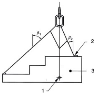
1. painopiste 2. suuri jännitys tässä jalassa 3. kuormitus P
