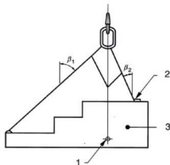
1. Środek ciężkości 2. Duże napięcie w tym cięgnię 3. Ładunek P
