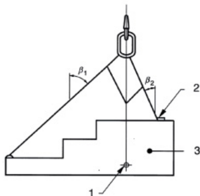
1. raskuskeskme 2. kõrge pinge selles jalas 3. koormus P
