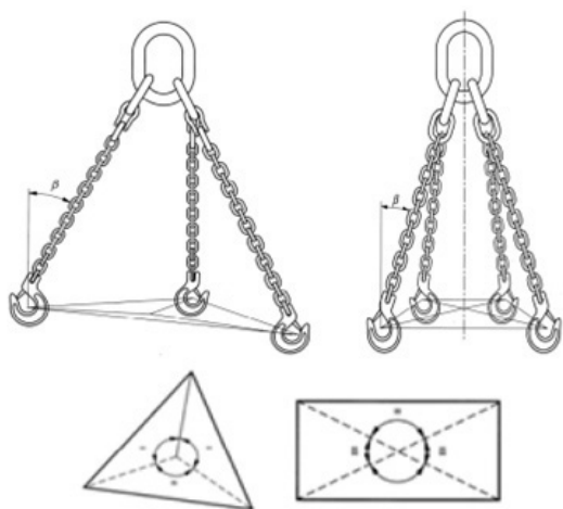
Koormuse sümmeetria
