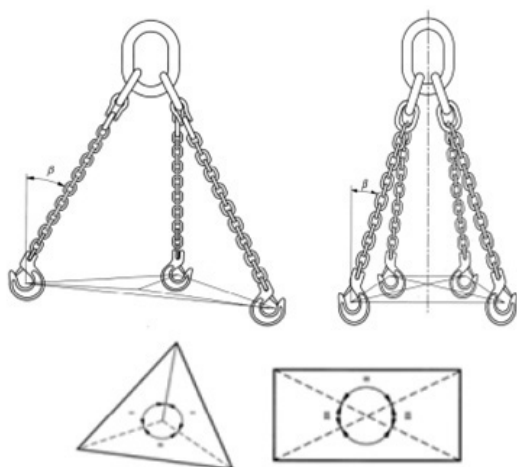
Lastningssymmetri
