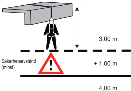
14 Rätvinkligt fall över kanten
