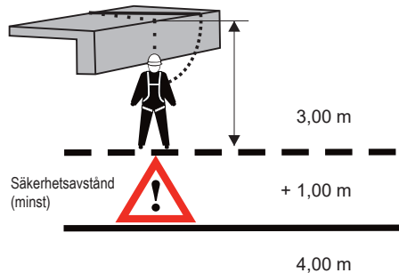
15 Sidofall över kanten
